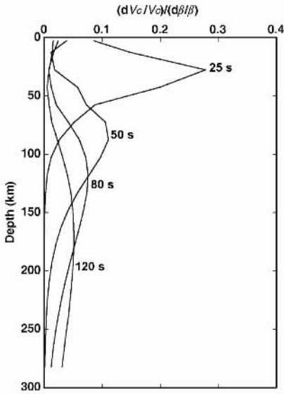
图 5 不同周期 Rayleigh 面波相速度 ( V_c ) 对深度方向上横波速度 ( \beta ) 的分辨核函数
